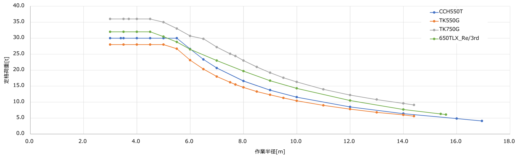
テレスコ4種性能比較 16mブーム
