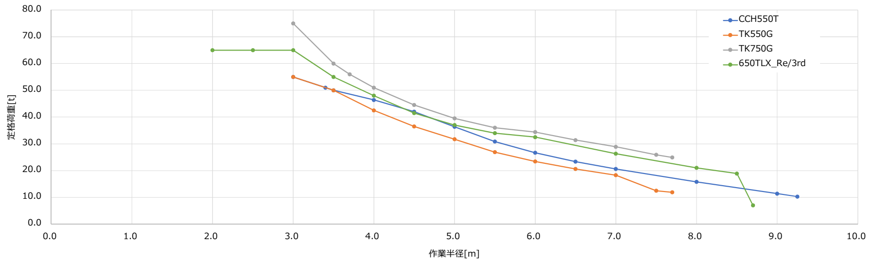
テレスコ4種性能比較 10mブーム
