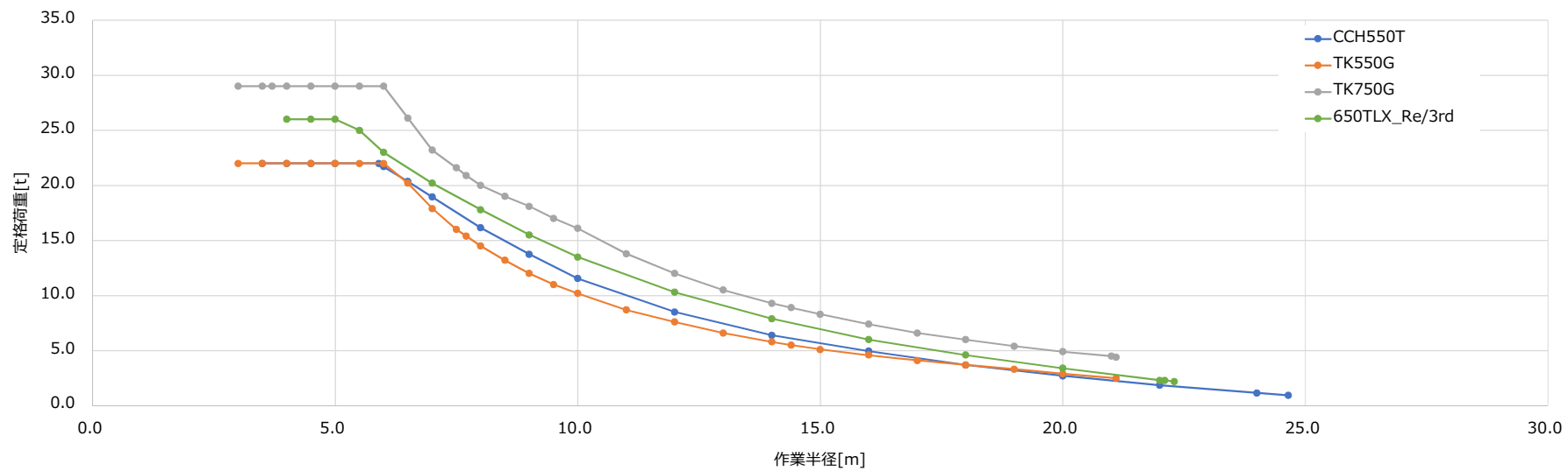
テレスコ4種性能比較 23mブーム
