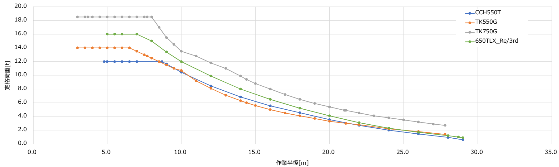
テレスコ4種性能比較 30mブーム
